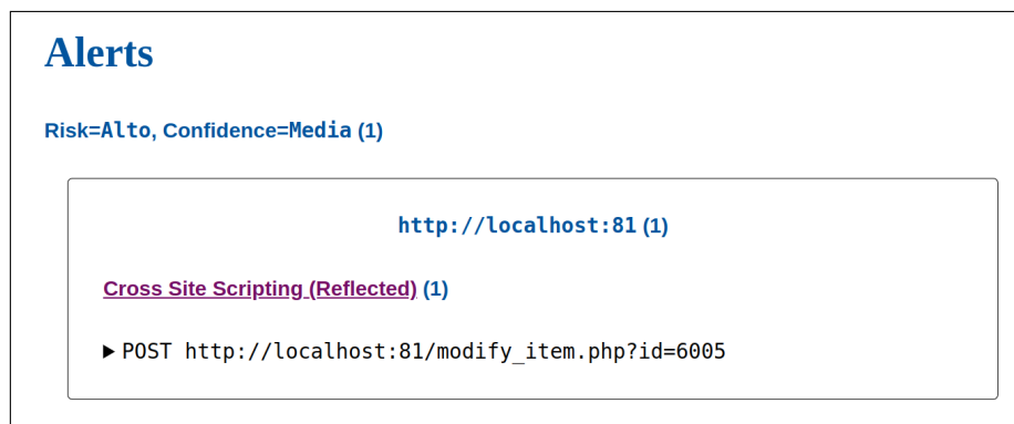
Figura 1: Errores de inyección detectados por ZAP.
